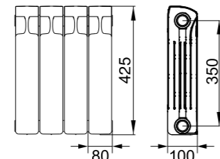
модель MONOLIT 350
