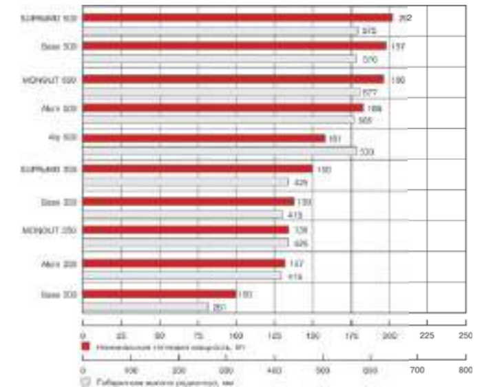
СРАВНЕНИЕ НОМИНАЛЬНОГО ТЕПЛООВОГО ПОТОКА И ГАБАРИТНОЙ ВЫСОТЫ СЕКЦИЙ РАДИАТОРОВ
