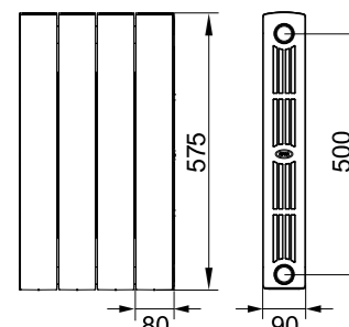
модель SUPReMO 500
